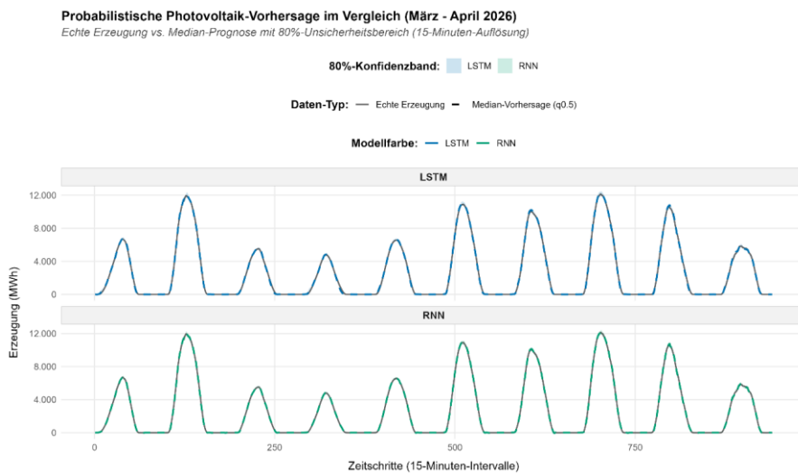
Abbildung 4.7: Probabilistische Photovoltaik-Vorhersage im direkten Architekturvergleich (Datensatz März-April 2026, 15-minütige Auflösung).
